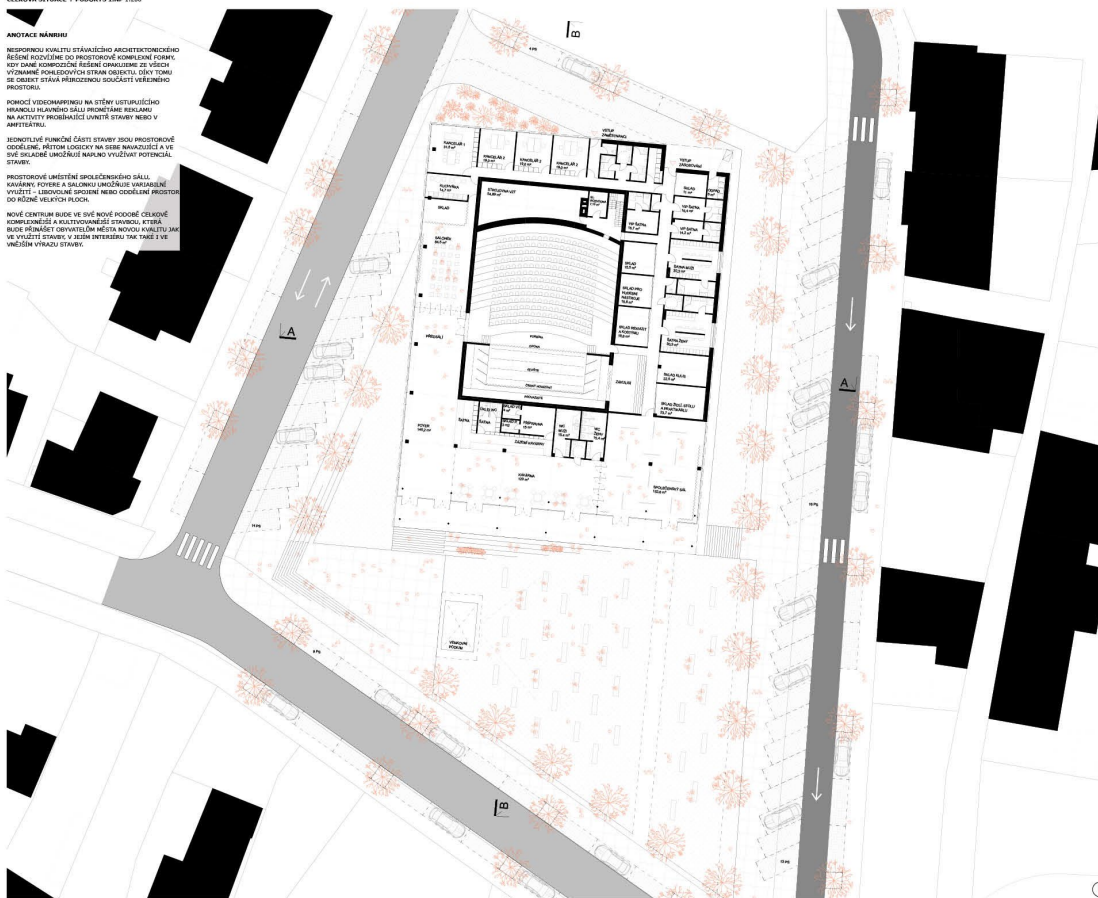
CELKOVÁ SITUACE - PŮDORYS LNP 1:200
